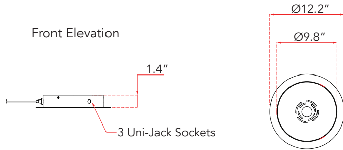
Top Elevation
