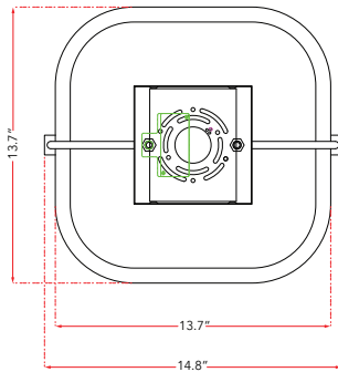
Top Elevation
